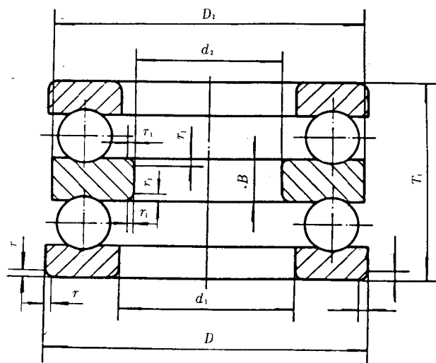
图 2 52000 型
