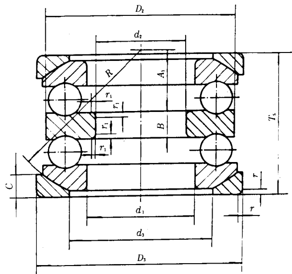
图 6 54000 U 型
