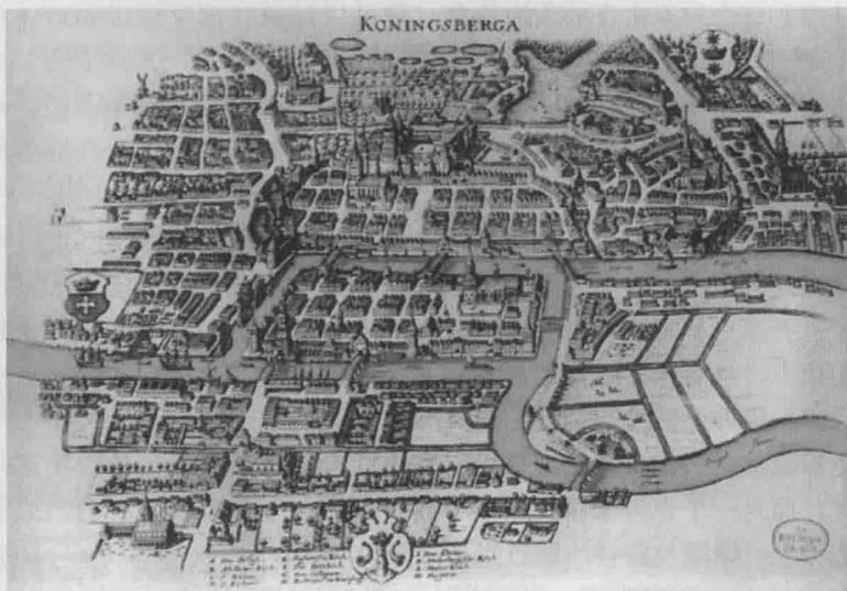
哥尼斯堡的七桥问题
