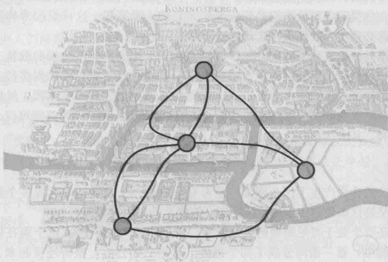
哥尼斯堡的七桥问题的图的表达
