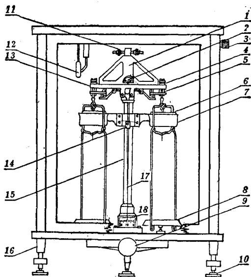
图 1-2 空气阻尼天平
