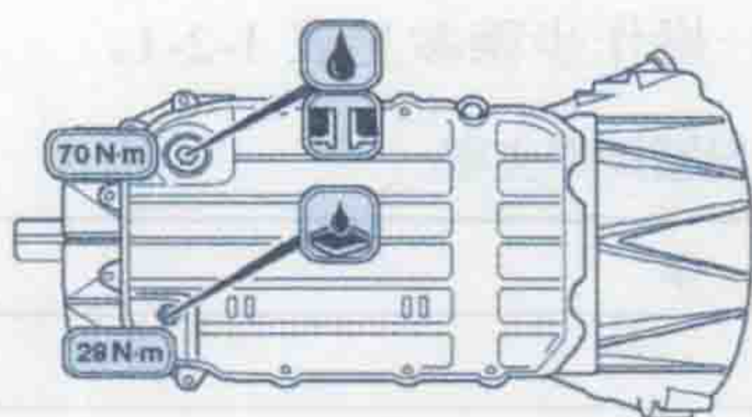
手动变速器
