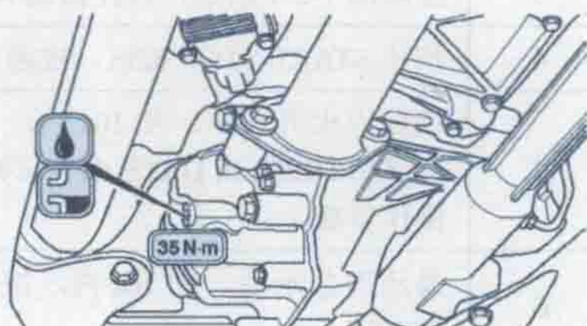
前桥差速器
