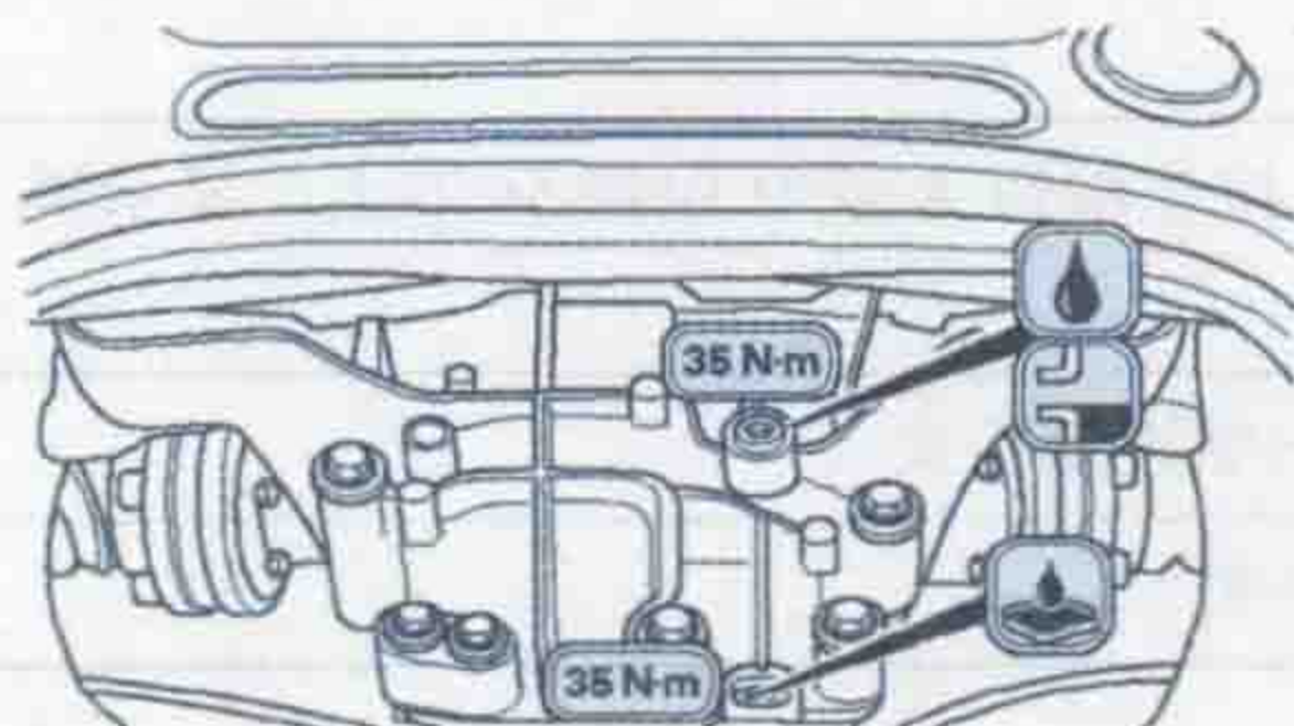
后桥差速器
