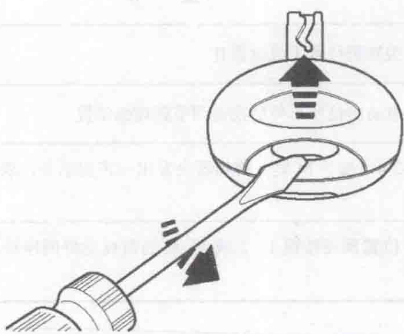
图 1-2-2 MINI 轿车遥控钥匙更换电池
