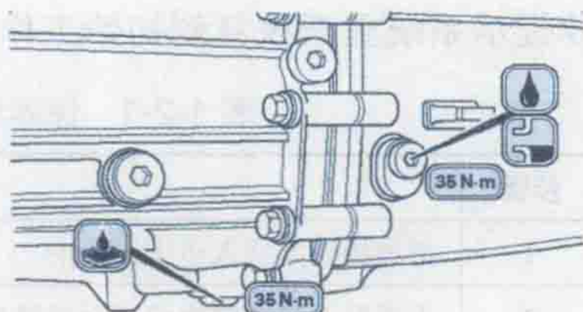
自动变速器
