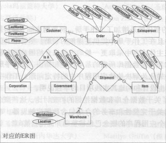
UML类图
