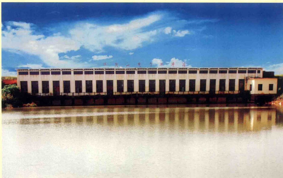
全省最大的电排站——康山锣鼓山电排站，装机容量7260千瓦。
