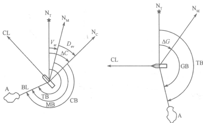
图 1-2 方位及其关系示意
