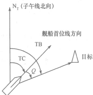
图 1-3 航向、方位和航向角之间的关系
