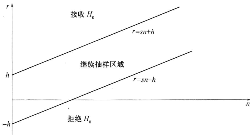
图 1.3 序贯概率比检验
