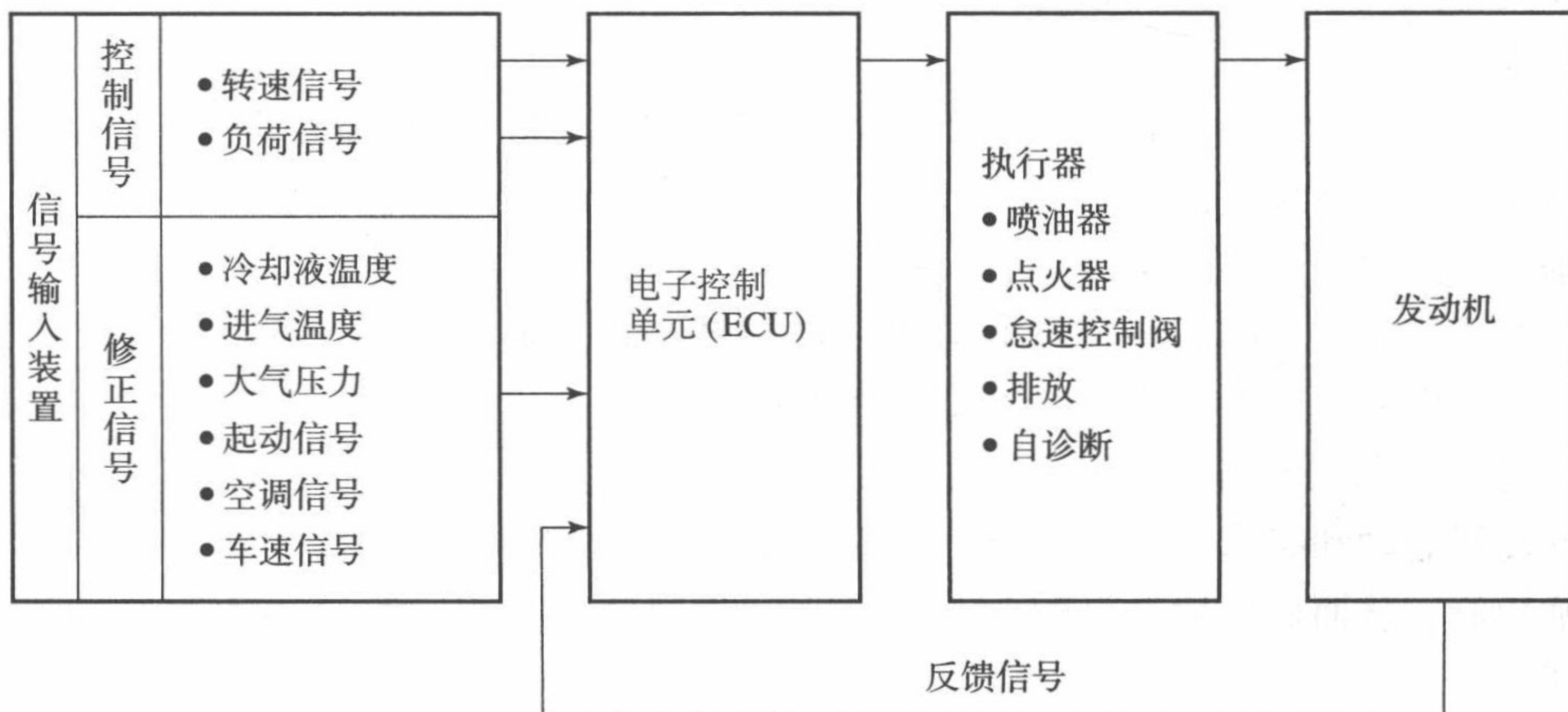
图 1-2 发动机电控系统工作原理的方框图
