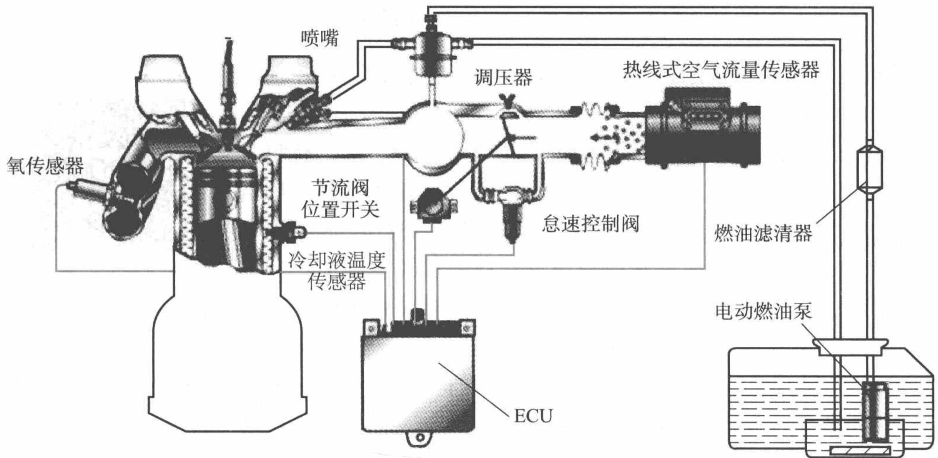
图 1-5 典型的汽油发动机电控系统的组成
