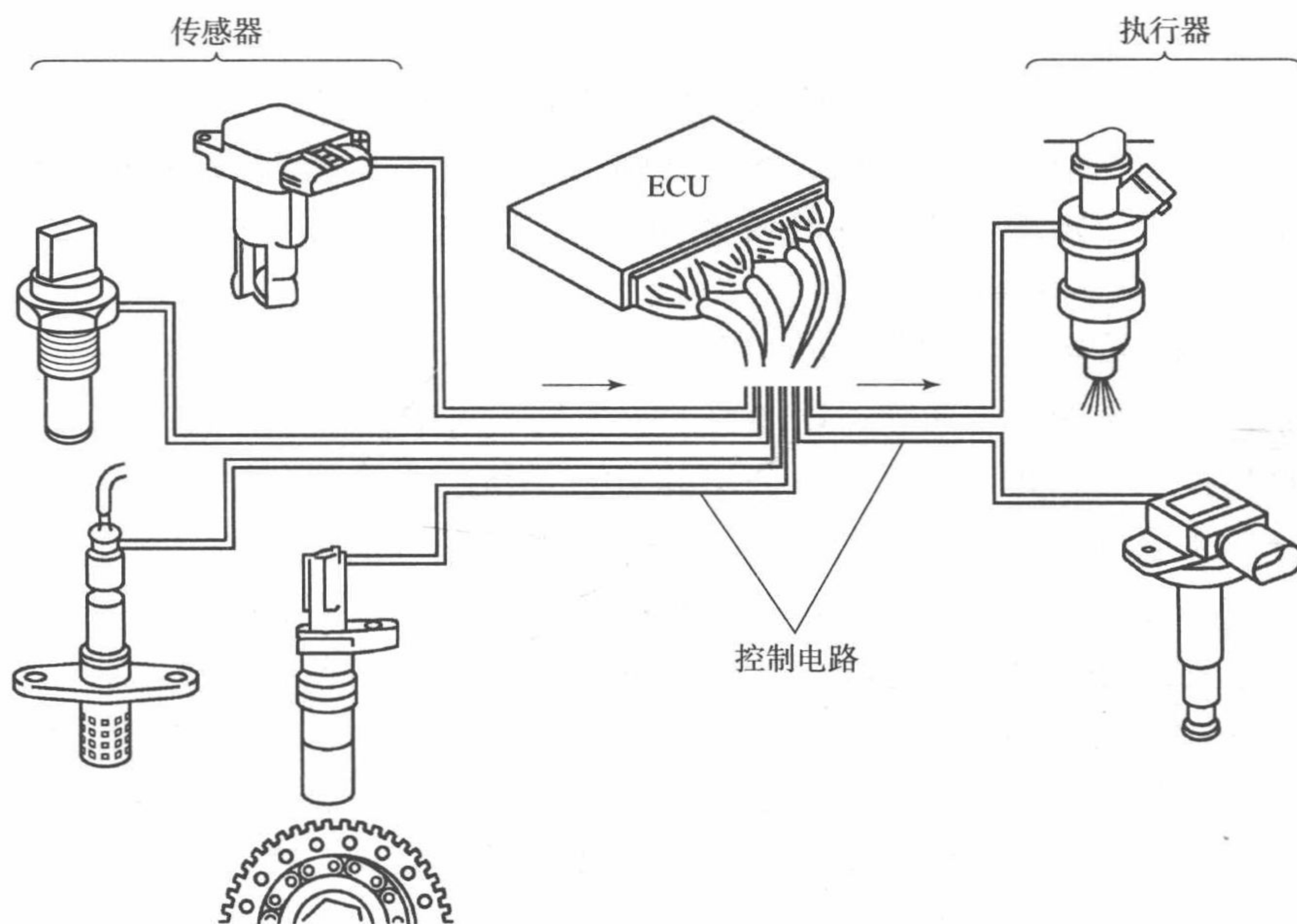
图 1-1 发动机电子控制系统的基本组成
