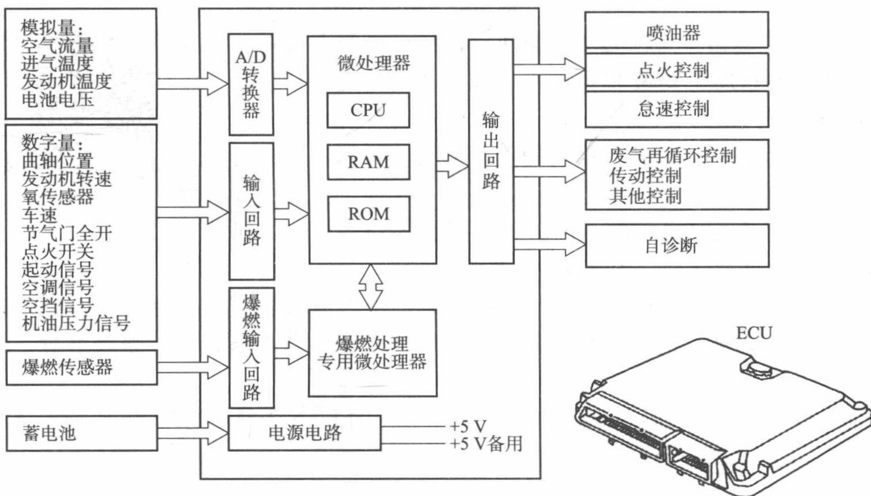
图 1-4 发动机 ECU 的功能
