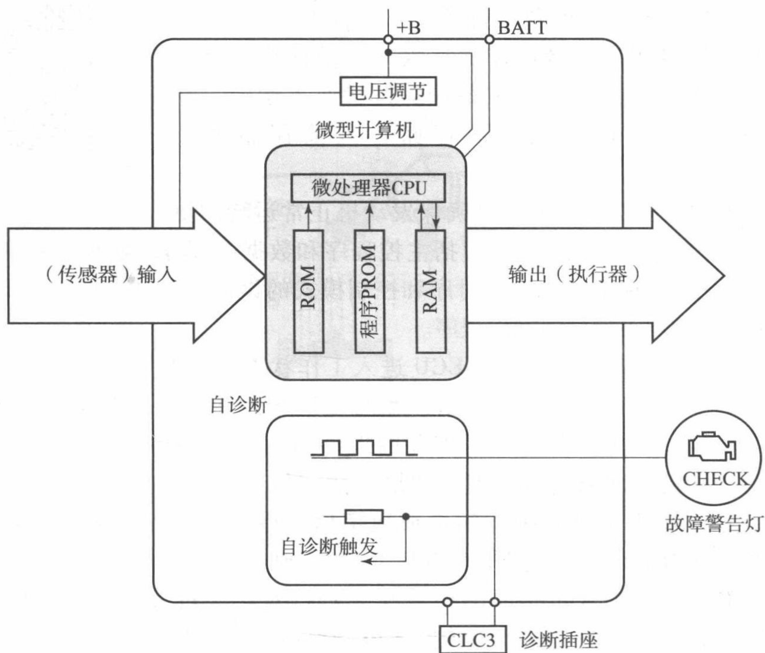
图 1-3 发动机 ECU 的内部组成
