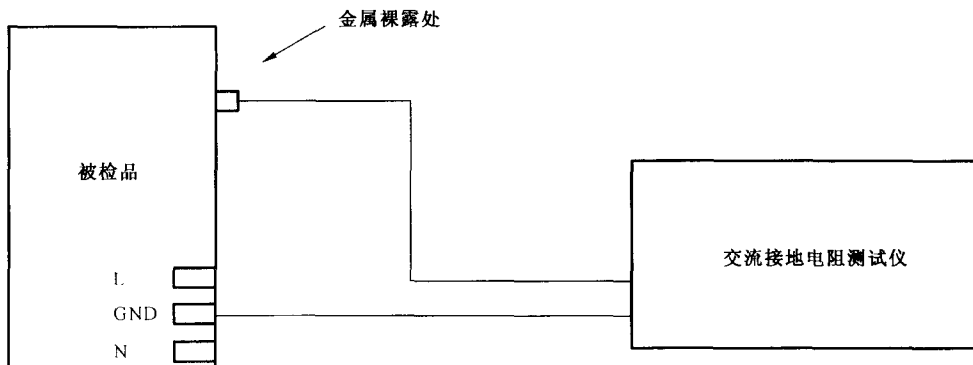
图 3 接地阻抗试验示意图
