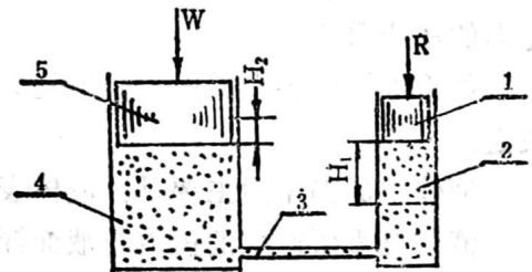
图 1-3 帕斯卡定律
