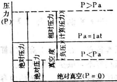
图 1-2 绝对压力和相对压力
