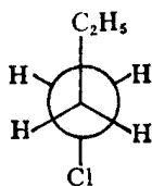
对位交叉
