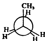
(II) 重叠式
