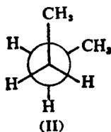
交叉式
