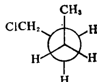
邻位交叉
