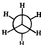
(II) 交叉式
