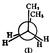
重叠式
