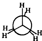
(I) 重叠式
