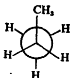
(I) 交叉式
