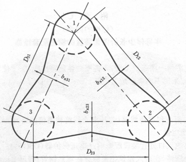
图 A3 三个等高消雷装置的保护范围
