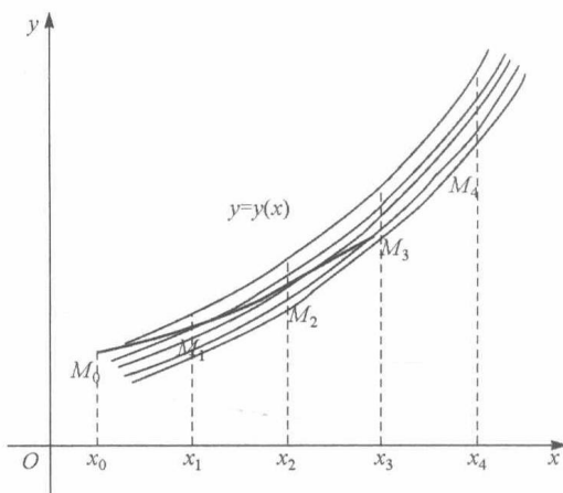
图 2.1 Euler 折线法
