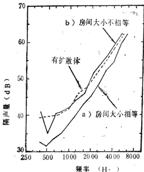
图2-1 3.5cm混凝土墙实测结果说明房间大小和扩散体的影响
