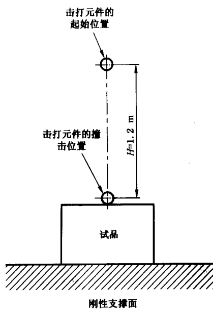
图 101 水平表面的撞击试验
