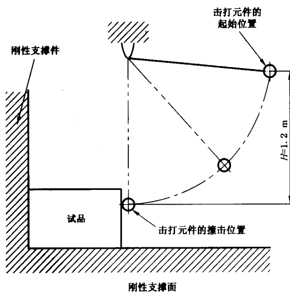
图 102 垂直表面的撞击试验
