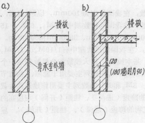
图 1-4 非承重外墙与平面定位线的关系
