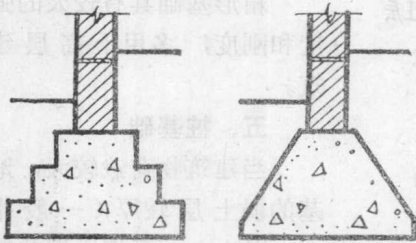
图 2-6 混凝土基础
