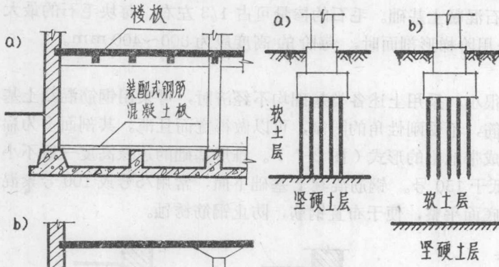
图 2-12 桩基础示意 a) 端承桩； b) 摩擦桩
