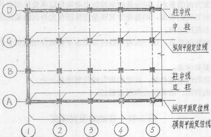
图 1-6 柱与平面定位线的关系
