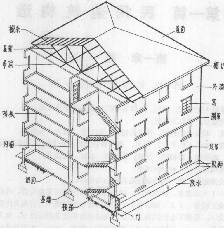
图 1-1 民用建筑的构造组成
