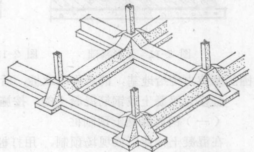
图 2-9 井格式基础
