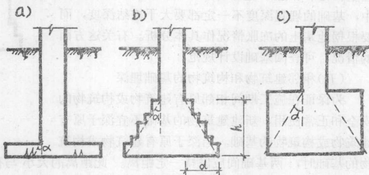
图 2-4 基础剖面与刚性角的关系
