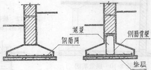
图 2-7 钢筋混凝土基础
