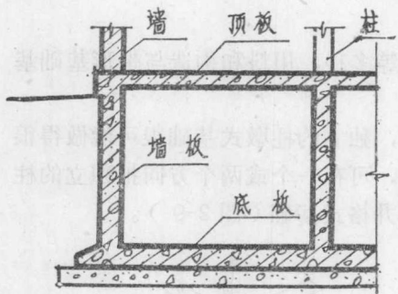
图 2-11 箱形基础
