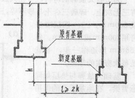
图 2-1 相邻基础的关系
