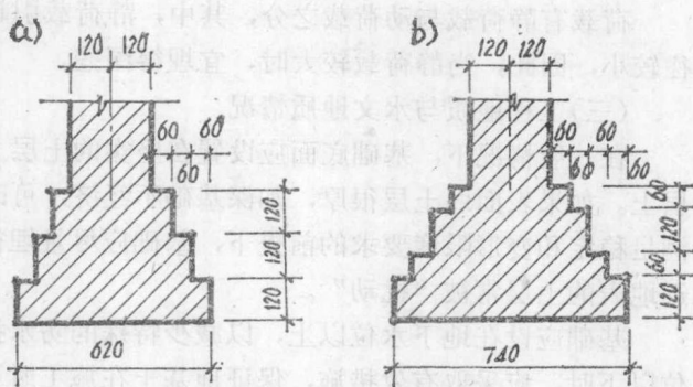
图 2-3 砖砌带形基础的大放脚
