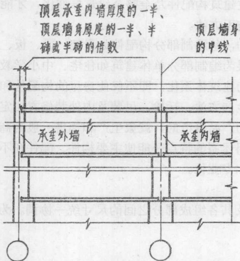
图 1-3 承重内、外墙与平面定位线的关系
