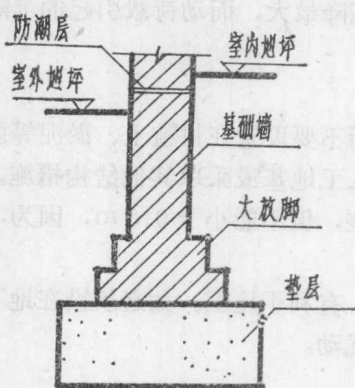
图 2-2 砖砌带形基础
