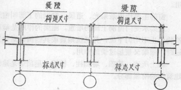
图 1-2 尺寸间的关系
