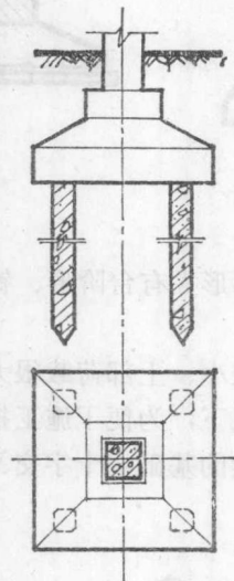
图 2-13 钢筋混凝土预制桩
