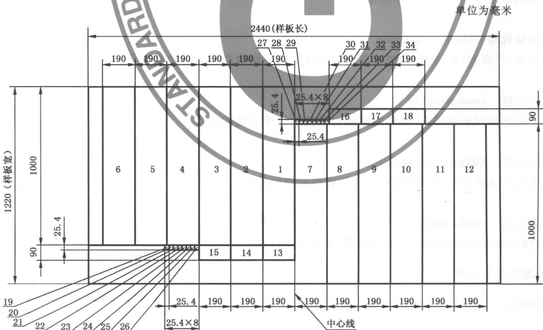
图 1 燃烧性能试件制备示意图
