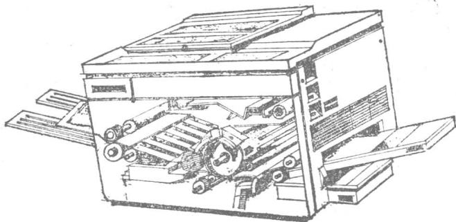
图表 2-1 Canon NP 复印过程示意
