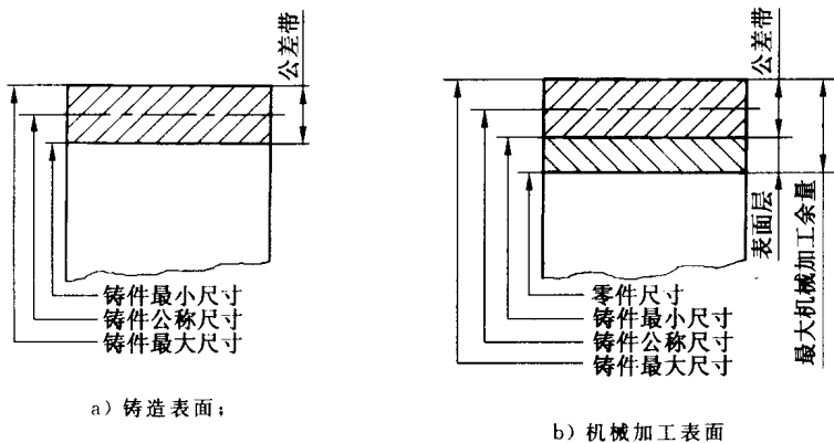
图 1-3 铸造毛面和机加工面的公差设置
