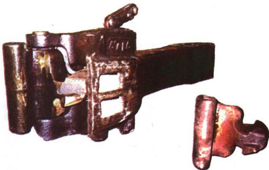
图 1-1 货车车钩铸钢件
