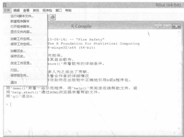
▲图 1-16 【文件】菜单
