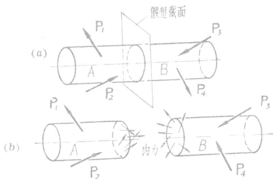
图 1-1 内力与截面法
