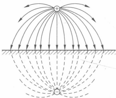
图 2-3 镜像法
