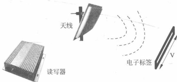
图 1-4 超高频 RFID 系统工作方式
