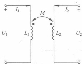
图 2-2 电感耦合图
