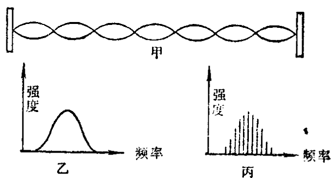
图 10 激光共振腔的选频作用
