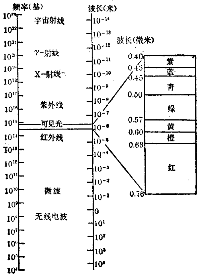
图 2 电磁波谱图
