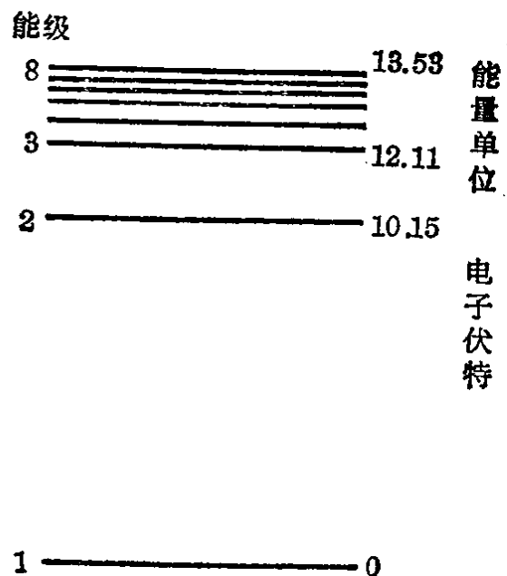
图4 氢原子能级图
