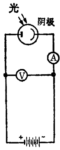
图 3 光电效应示意图
