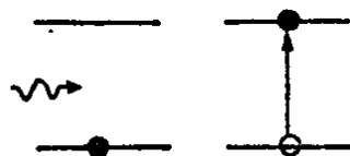
图6 受激吸收
