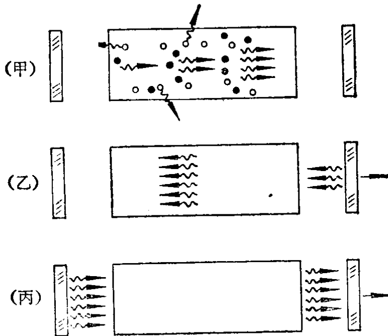
图 9 激光共振腔的反馈作用
