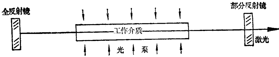
图 8 激光器示意图
