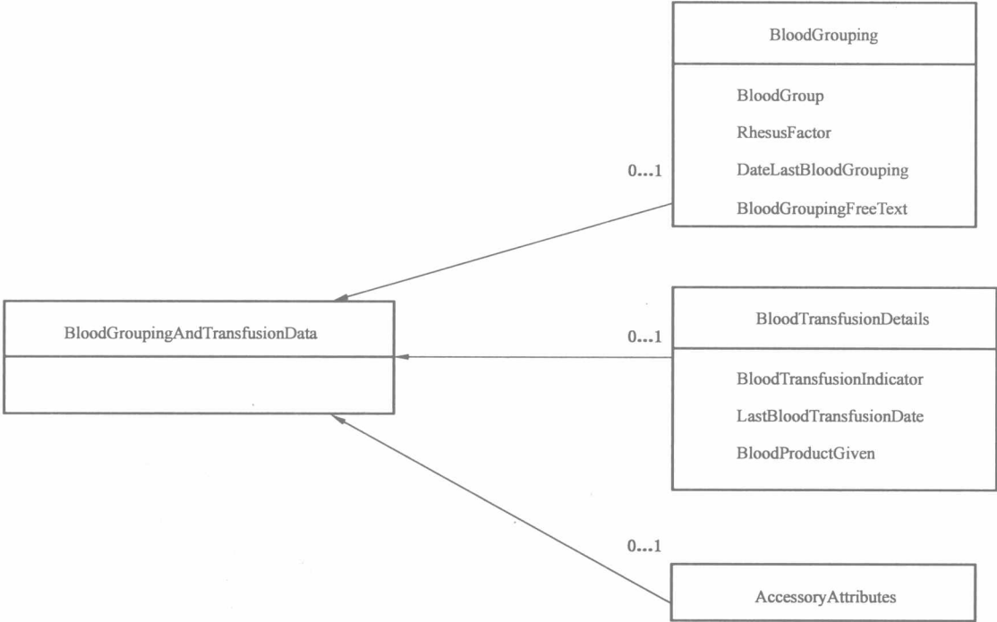
图 5 “BloodGroupingAndTransfusionData”的结构
