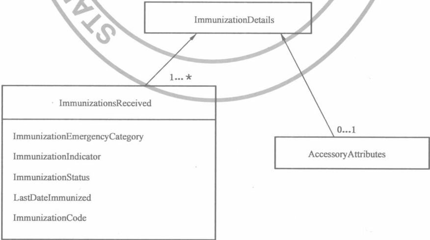
图 4 “ImmunizationDetails”的结构
