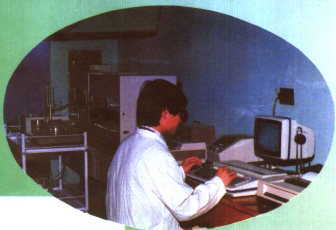
用于微量元素分析的双光束原子吸收分光光度计。
