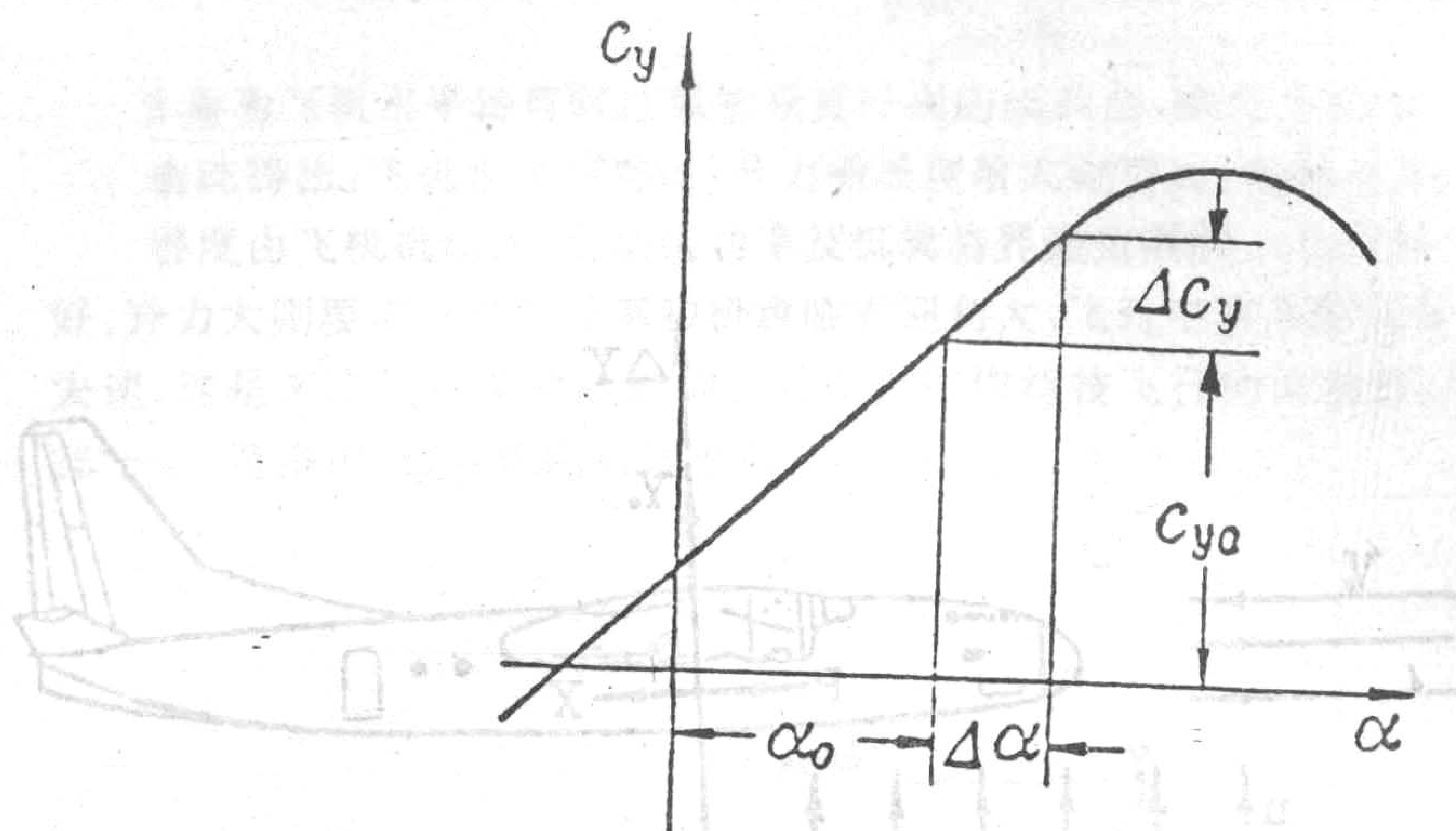
图 1—6 升力系数曲线
