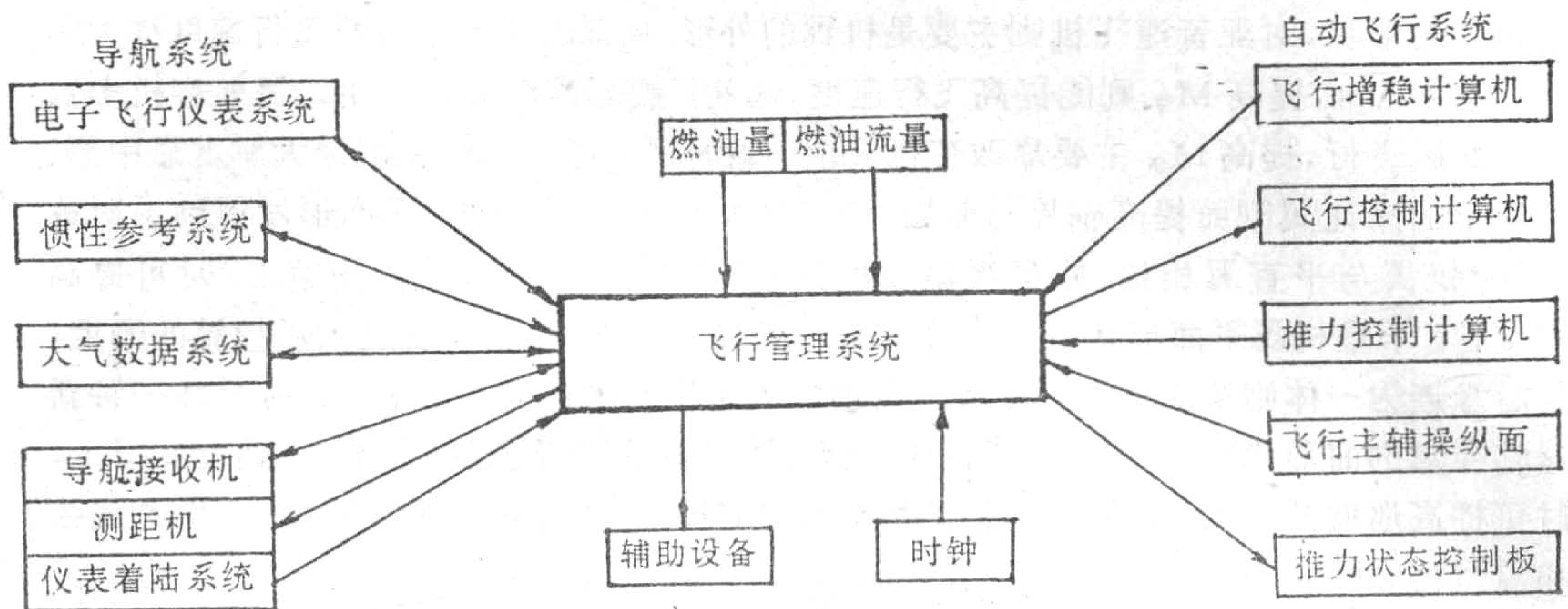
图 0—3 飞行管理系统与其它设备的交联
