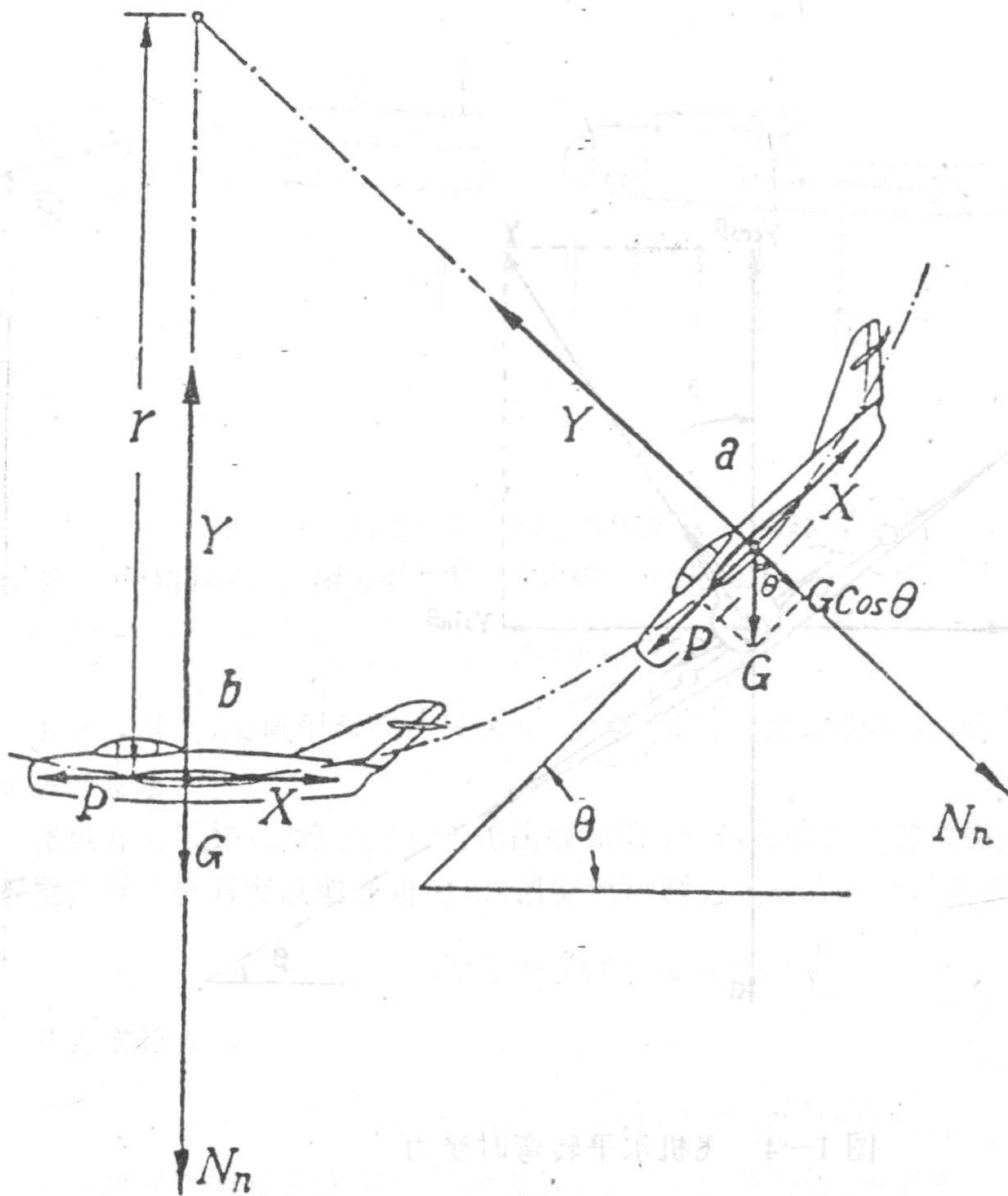
图 1—3 飞机在垂直平面内曲线飞行受力
