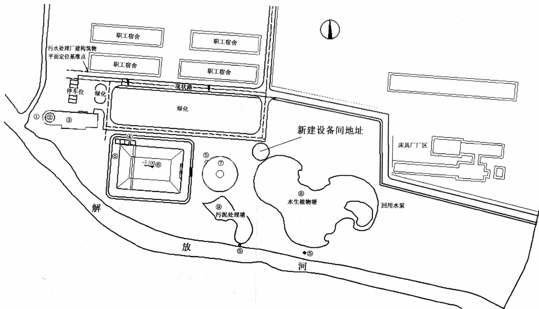
图 5-9 南京陆军指挥学院污水处理回用总平面布置图
