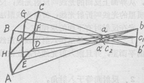
图（1—1）象散光束
