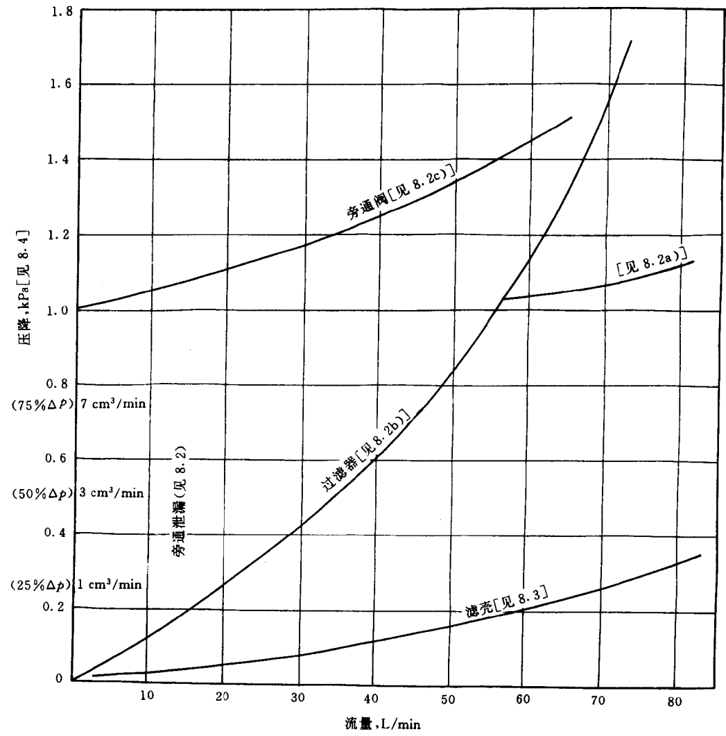
图 2 对于一个带有内装旁通阀的过滤器的压降流量曲线和旁通泄漏流量的典型表达
