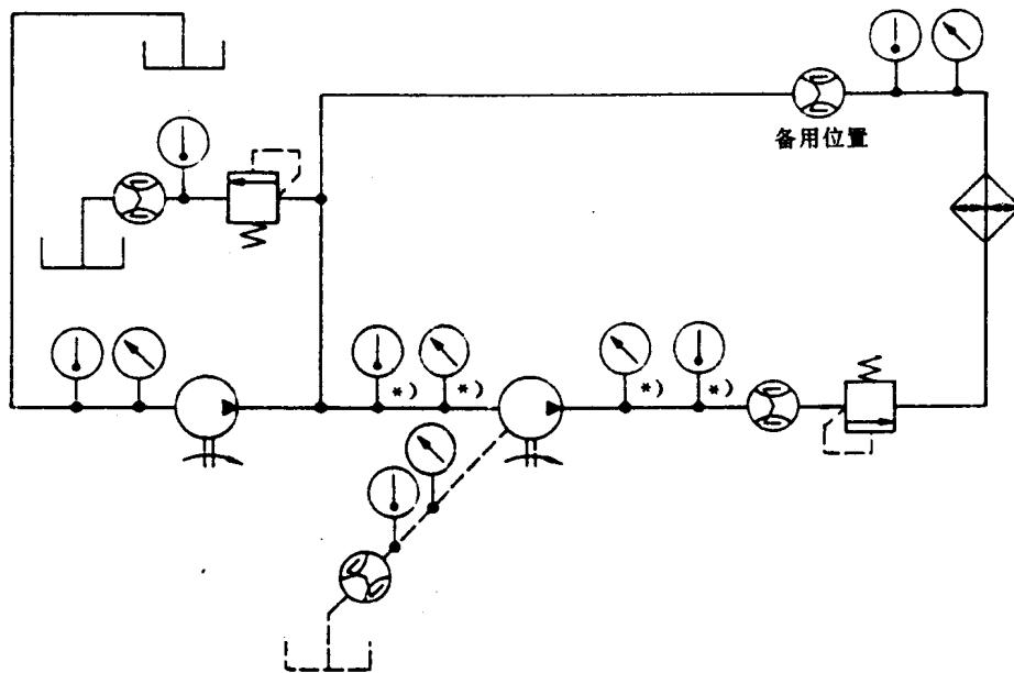
图 2 泵元件的试验回路(闭式回路)
