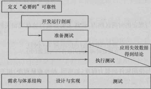
图 1.3 软件可靠性工程过程框架(Musa) [2]
