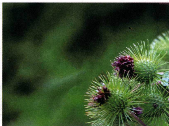
图 1-13 处理后效果
