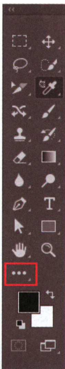
图 1-2 编辑工具栏
