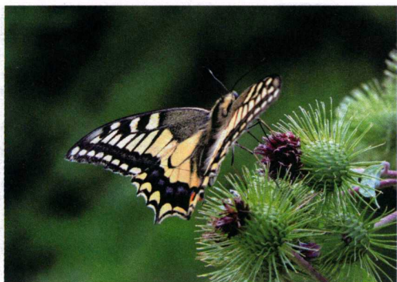
图 1-12 原始图片
