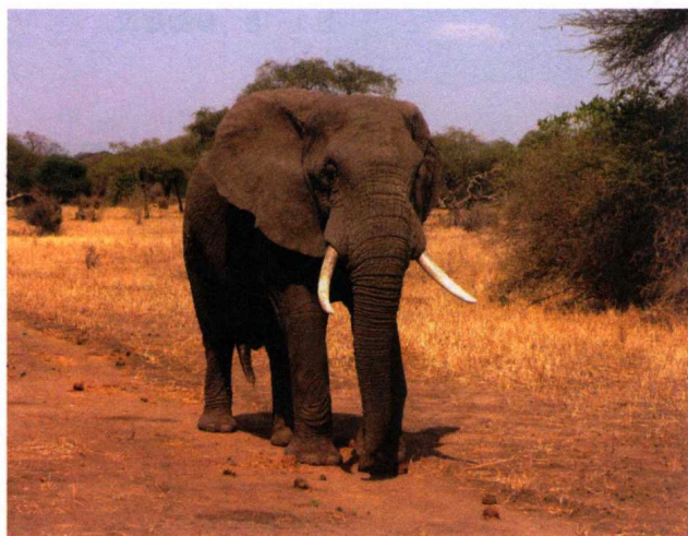
图 1-16 大象原图
