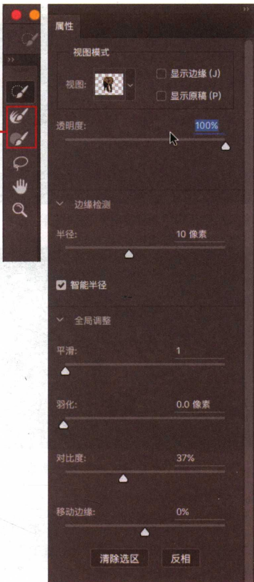
图 1-18 参数建议
