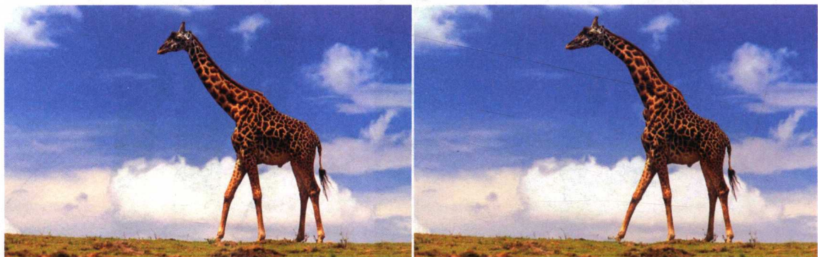
图 1-20 前后对比图
