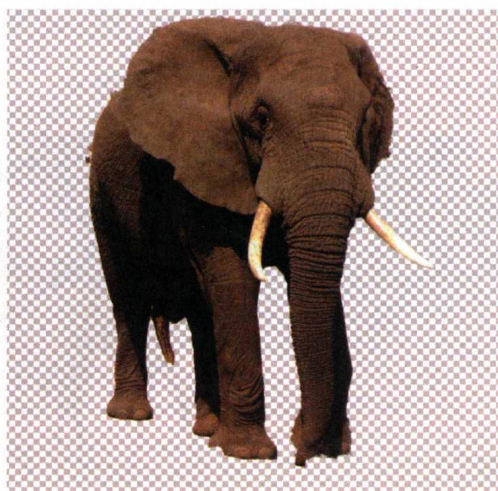
图 1-17 大象抠像
