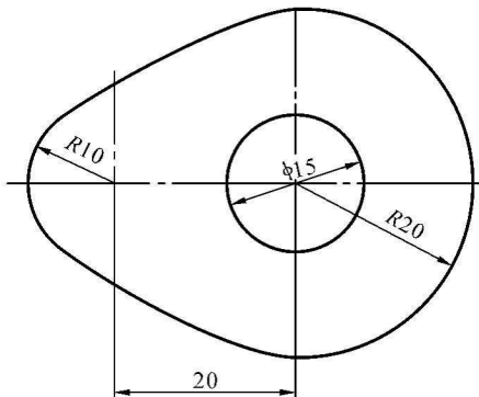
图 1-24 垫片零件 2
