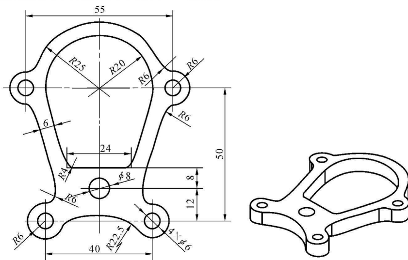
图 2-1 垫片尺寸
