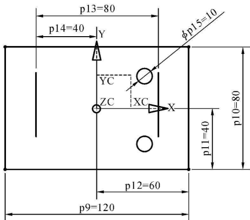
图 1-9 绘制两个圆
