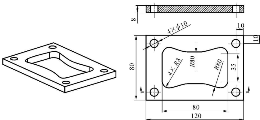
图 1-1 盖板尺寸
