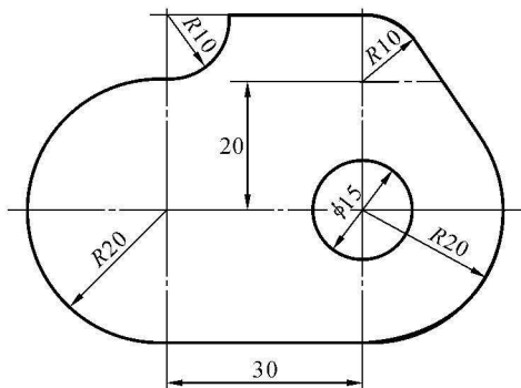
图 1-23 垫片零件 1
