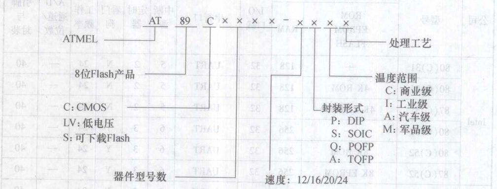
图 0-1 AT89 系列单片机型号含义
