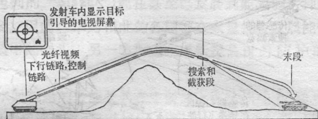
图1.2 光纤控制的战术导弹
