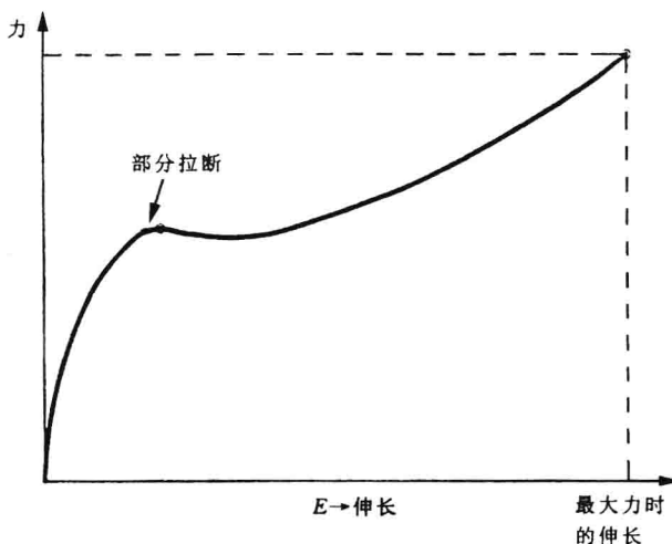
图 3 涂覆织物部分拉断
