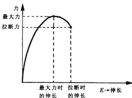
图 2 拉断瞬间的拉伸力
