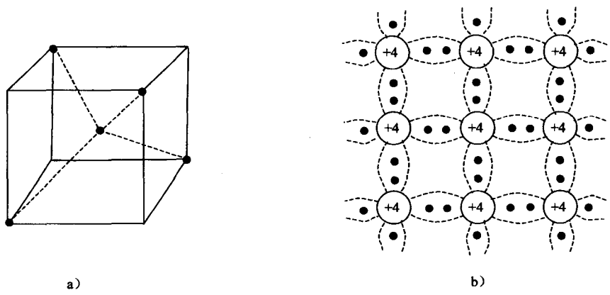
图 2-2 硅和锗的共价键结构 a) 四面体结构 b) 二维晶格结构示意图
