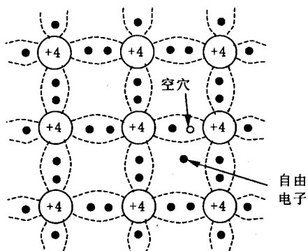
图 2-3 本征激发电子-空穴对
