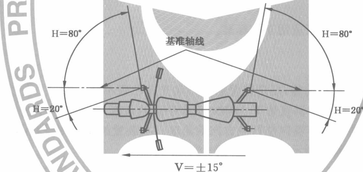
图 3 转向信号灯的类别和光分布最小角
