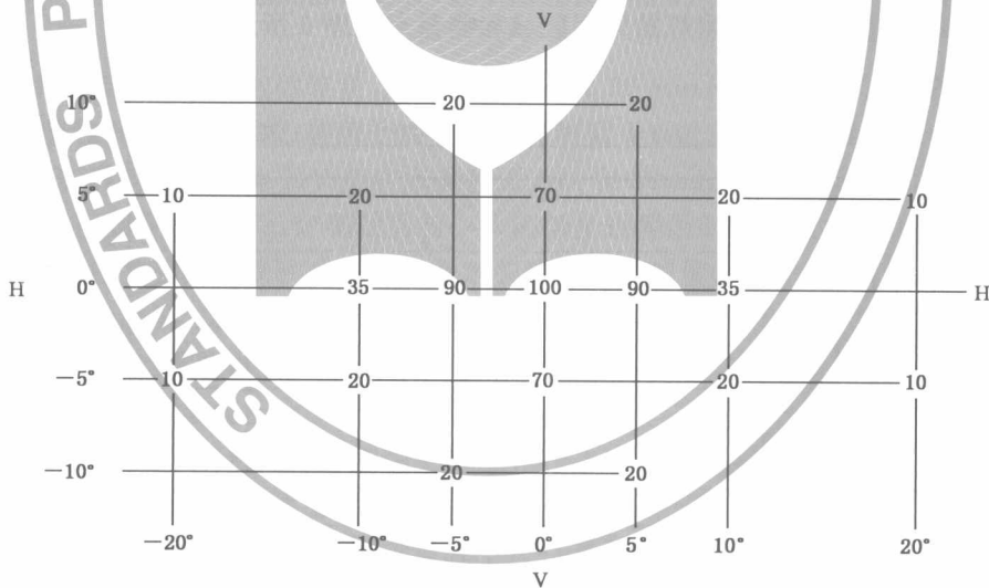
图 5 发光强度分布范围
