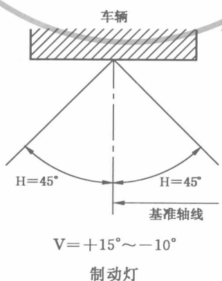
图 4 制动灯的光分布最小角
