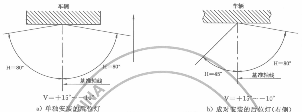
图 2 后位灯的类别和光分布最小角
