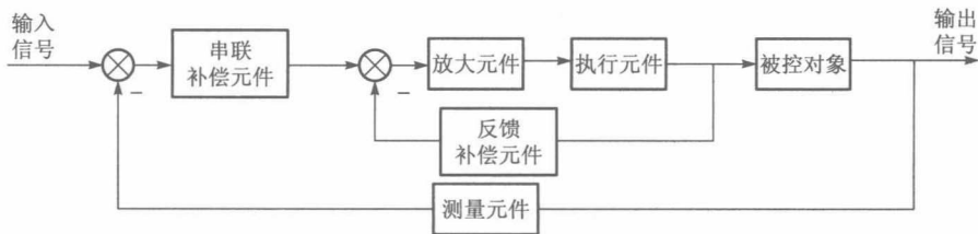
图 1-5 自动控制系统的基本组成
