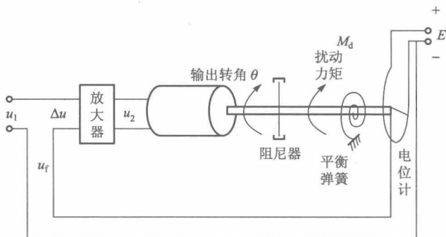
图 1-4 闭环控制系统
