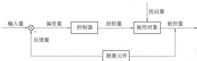
图 1-3 闭环控制系统示意图
