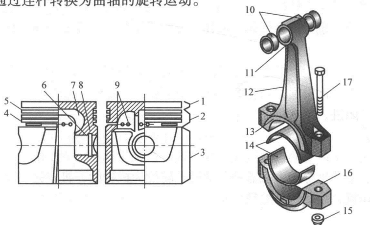
图 1-2 活塞与连杆结构
