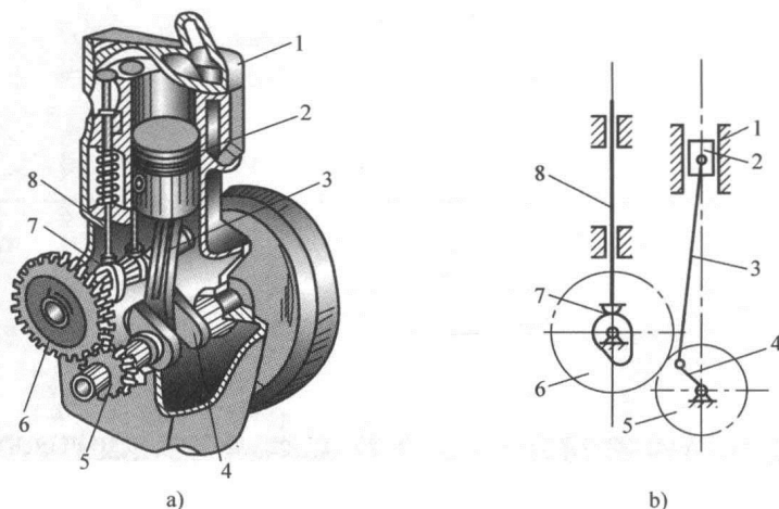
图 1-1 内燃机机构
