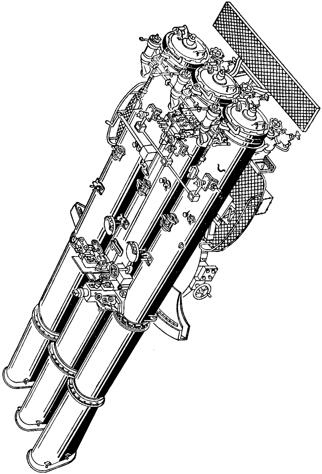
图1-13 驱逐舰上的鱼雷发射管
