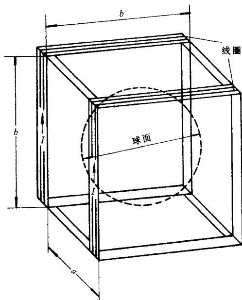
图 7 亥姆霍兹线圈示意图
