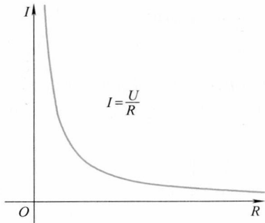
图 1.4 电流强度越来越小
