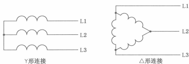
图 4 三相三线制
