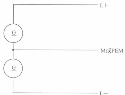
图 7 三线制
