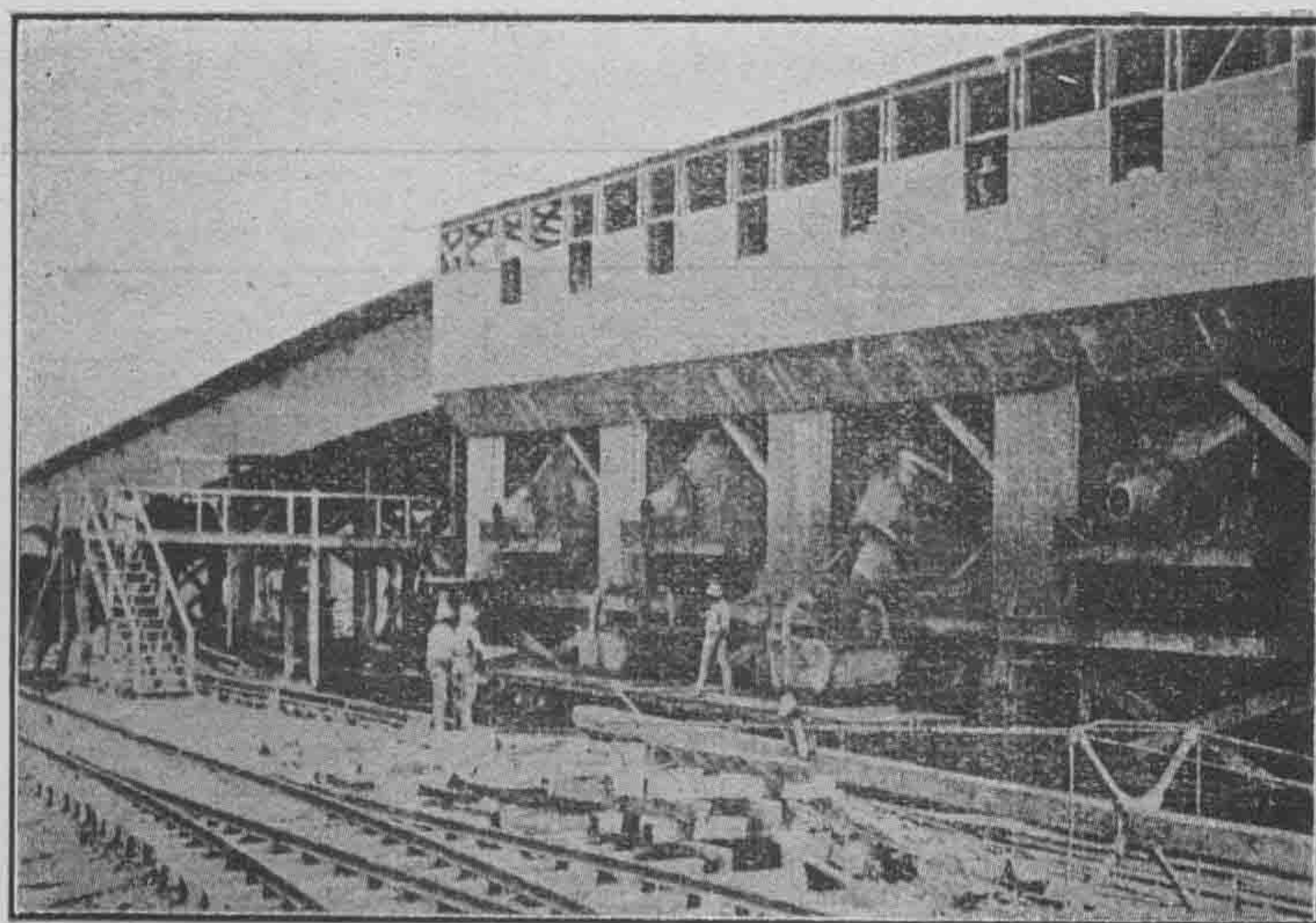
嘉 敦 閘 和 石 土 之 機 器
