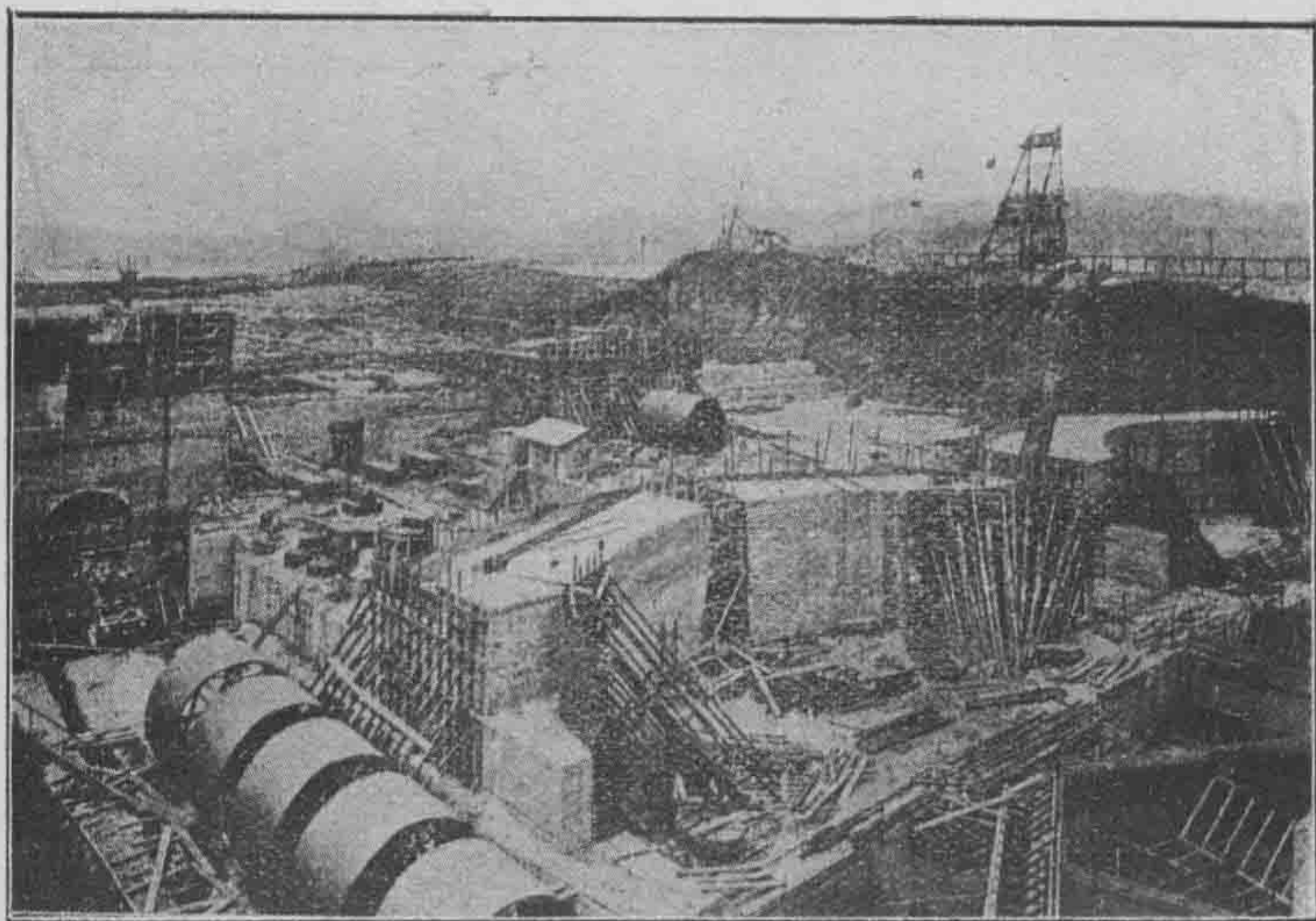
嘉敦閘東面之前灣及土臺
