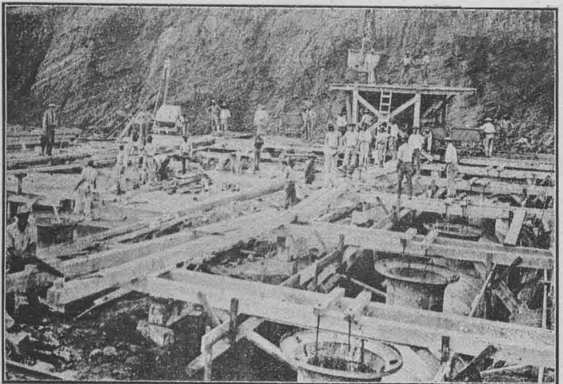
渠水及面橫之閘爾加米羅得比
