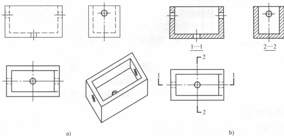
图 1-10 水槽的全剖面图
