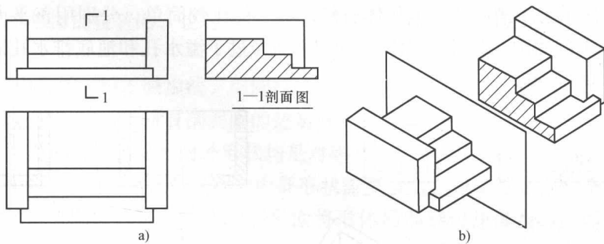
图 1-8 台阶剖面图的形成
