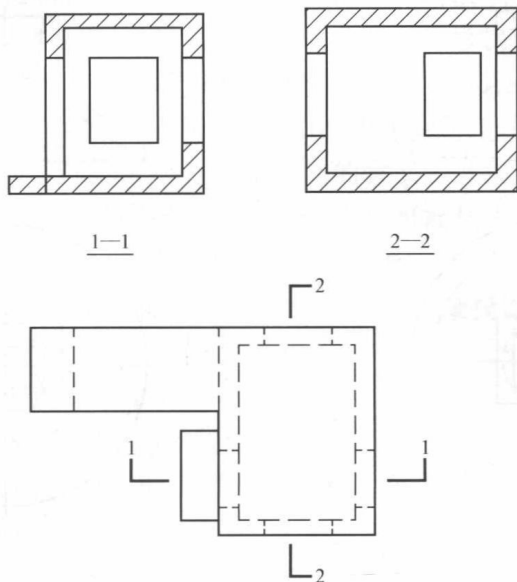
图 1-9 剖面图及其剖切符号
