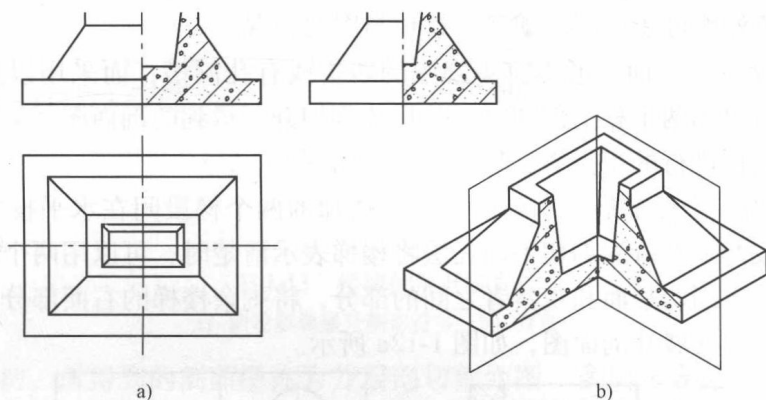
图 1-11 杯形基础的半剖面图
