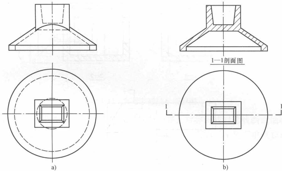
图 1-7 圆锥形薄壳基础的视图和剖面图
