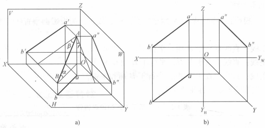
图 1-6 一般位置直线的投影 a) 直观图 b) 投影图
