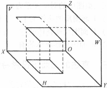
图 1-4 面的投影
