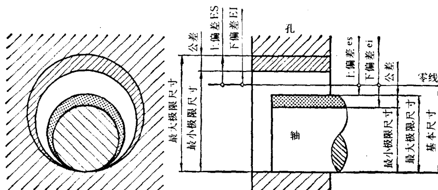
图 1 公差与配合的示意图
