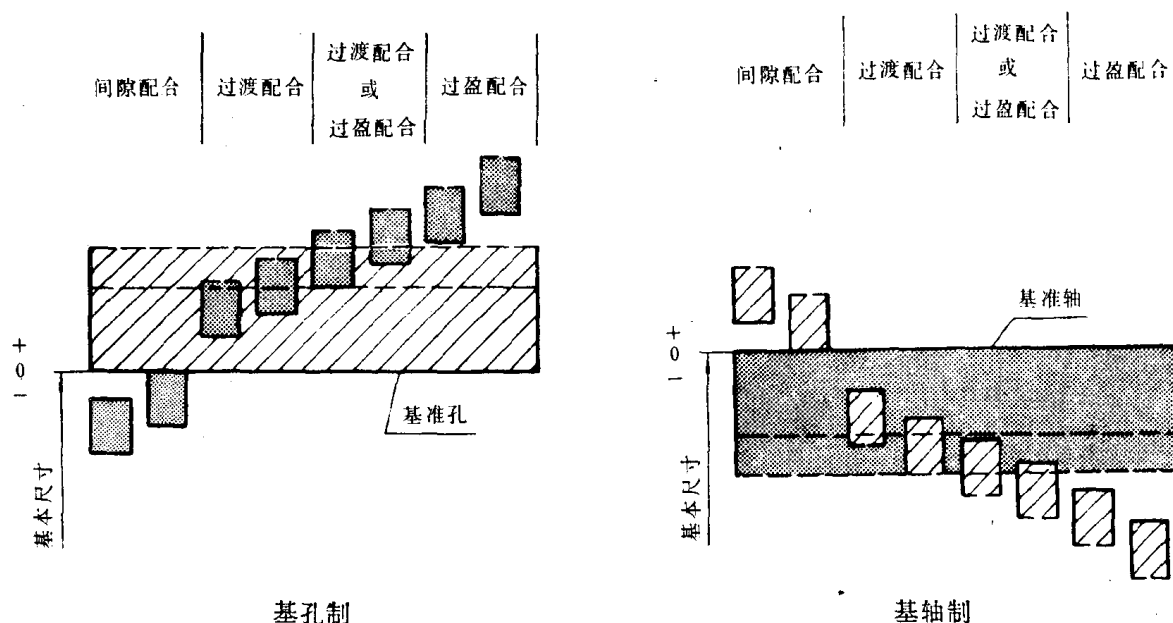
图7 基孔制和基轴制
