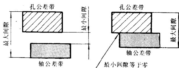
图4 间隙配合
