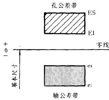
图 2 公差带图
