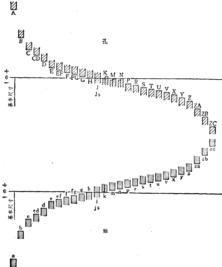
图 3 基本偏差系列
