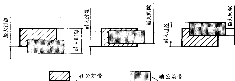
图6 过渡配合
