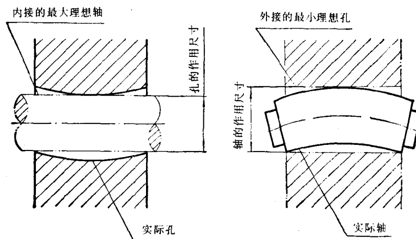
图8 孔或轴的作用尺寸
