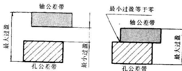
图5 过盈配合
