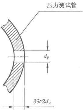
图 C.2 压力测试孔
