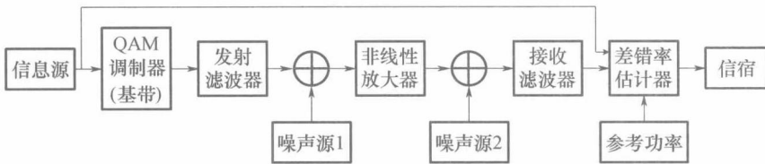
图 1-3-1 通信系统仿真简化模型
